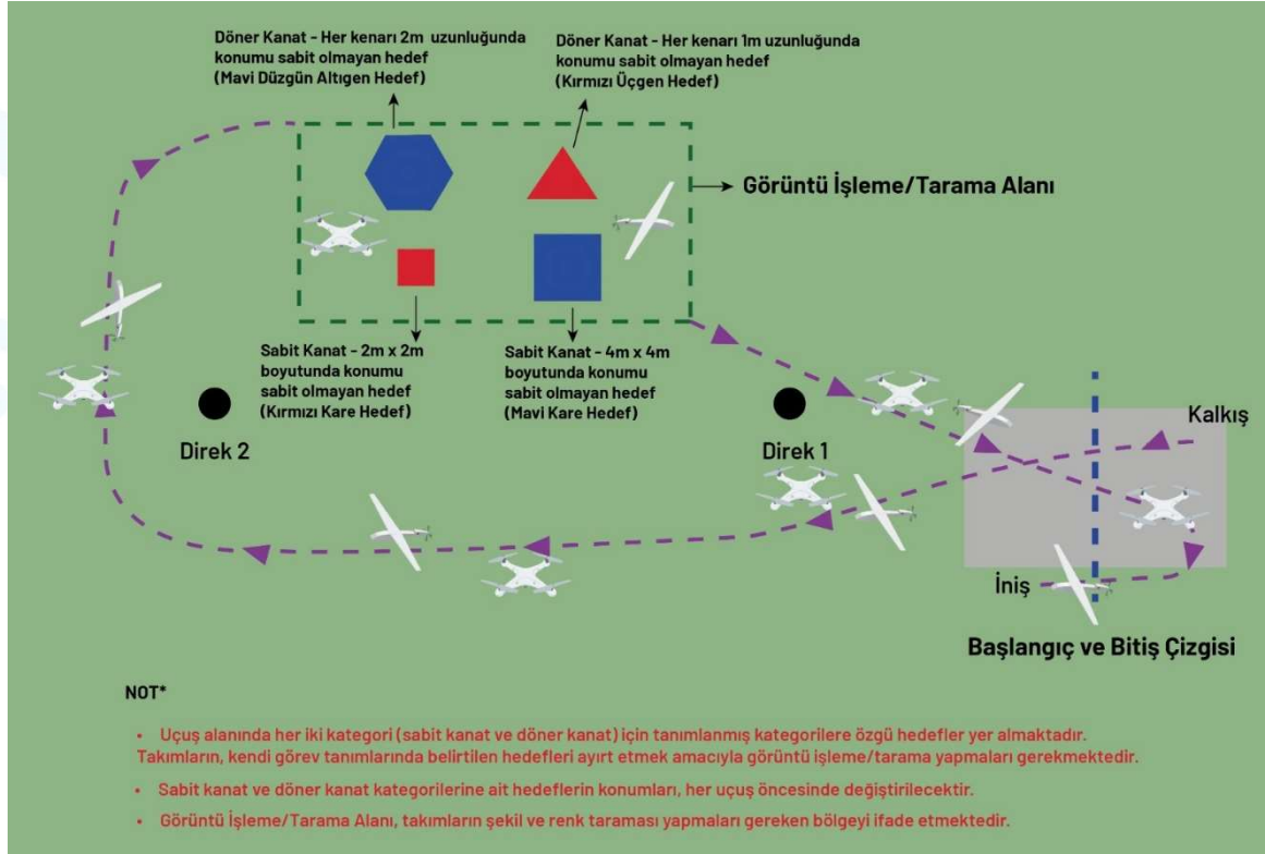
Şekil 3. Uluslararası İHA Yarışması İkinci Görev Uçuş Güzergâhı
