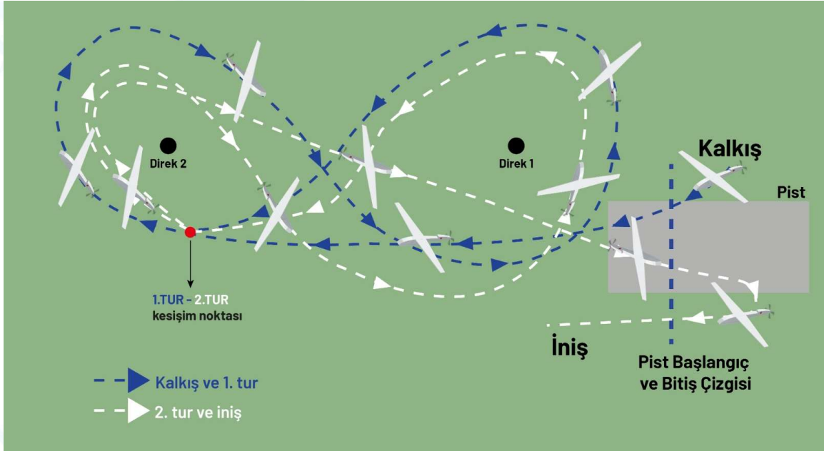
Şekil 4. Liseler Arası İHA Yarışması Sabit Kanat Kategorisi Birinci Görev Uçuş Güzergâhı
