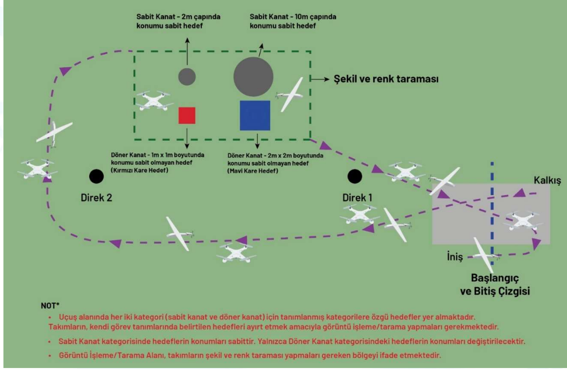
Şekil 9. Liseler Arası İHA Yarışması İkinci Görev Uçuş Güzergâhı
