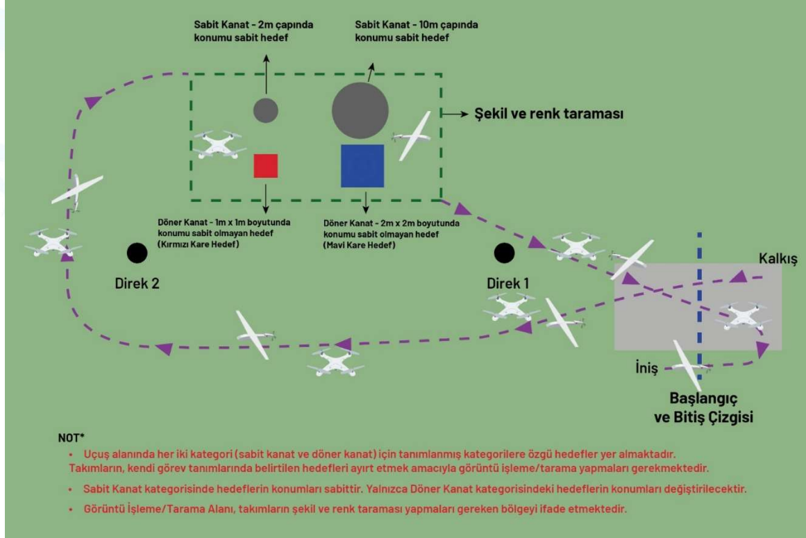
Şekil 5. Liseler Arası İHA Yarışması İkinci Görev Uçuş Güzergâhı
