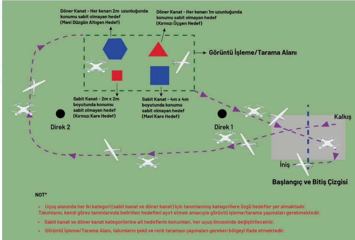
Şekil 7. Uluslararası İHA Yarışması İkinci Görev Uçuş Güzergâhı
